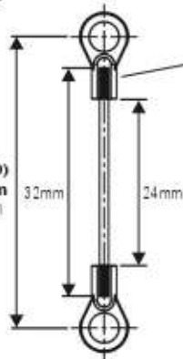
Linkage rod(D) Approx. 42mm 連桿 (D) 約42mm
