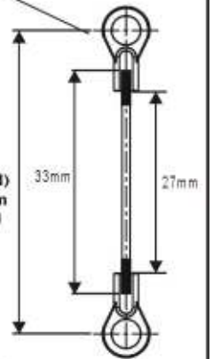
Linkage rod(N) Approx. 45mm 連桿 (N) 約45mm
